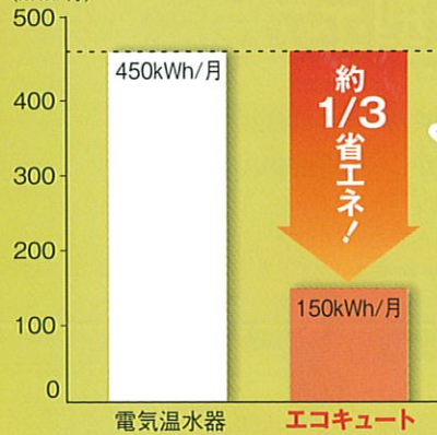
■電気温水器とエコキュートの電気使用量比較 (kWh/月)
